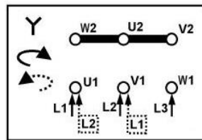
Sternschaltung
